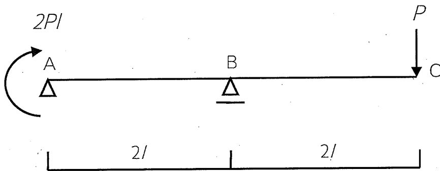
図1 張り出し梁
