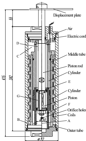
MR 緩衝器
