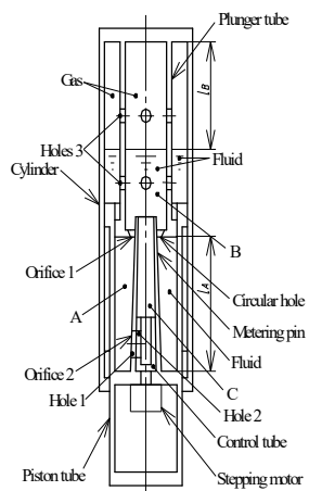
バイパスオリフィス式油圧緩衝器
